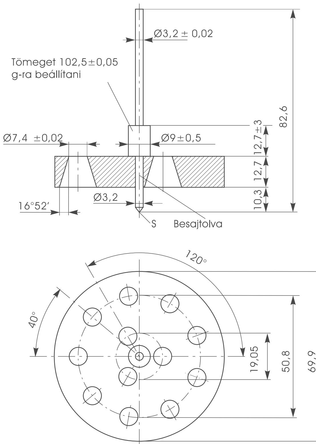
4. ábra: Penetrométer
